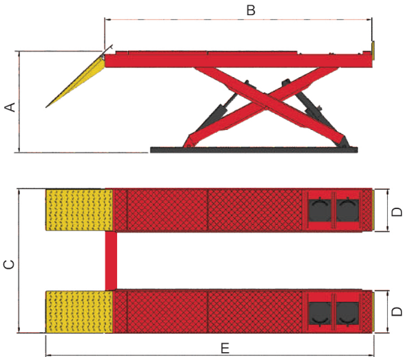
AX-12A
